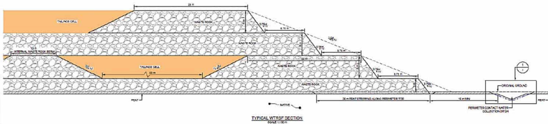
Figure 4 Halde à stériles – Coupe transversale
